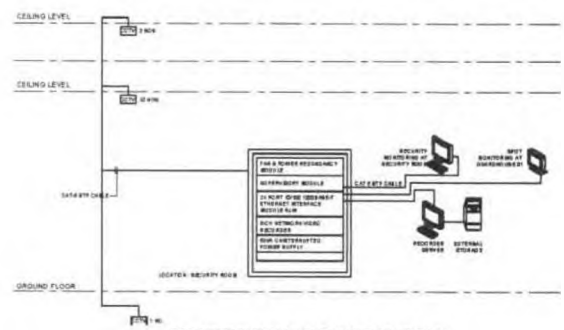
SECURITY SYSTEM SCHEMATIC DIAGRAM SCALE: N.T.S.
